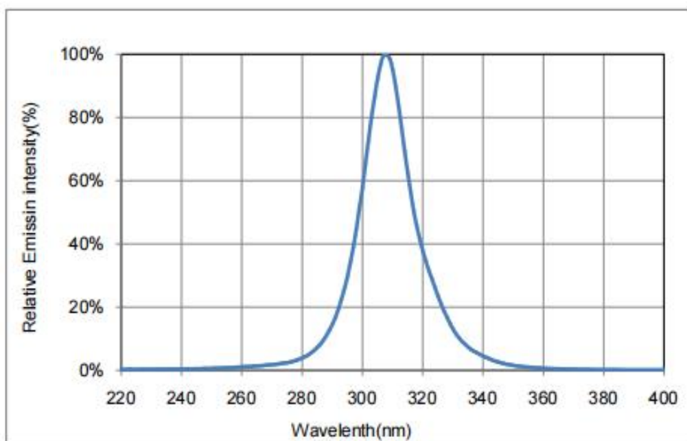
Fig.5-Spectrum Distribution 光谱分布特性曲线
