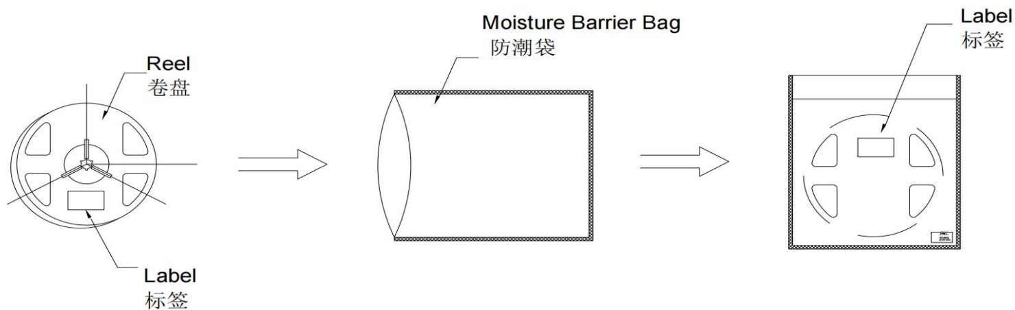
Fig.2-4 Moisture Resistant Packing Process 防潮包装过程
